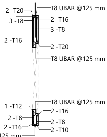
2 SECTION(REINF) 1 : 50
