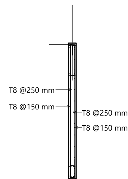
3 SECTION(REINF) 1 : 50
