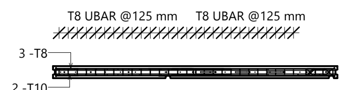
6 SECTION(REINF) 1 : 50
