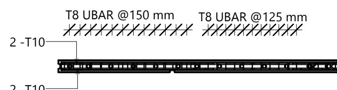
4 SECTION(REINF) 1 : 50
