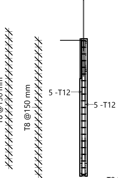
1 SECTION(REINF) 1 : 50
