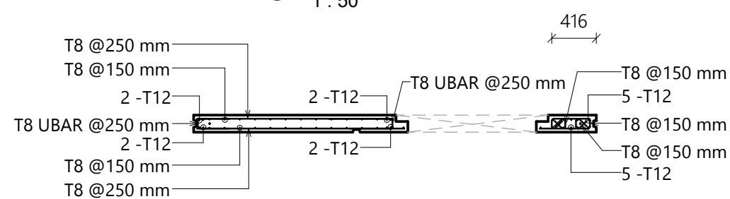
5 SECTION(REINF) 1 : 50
